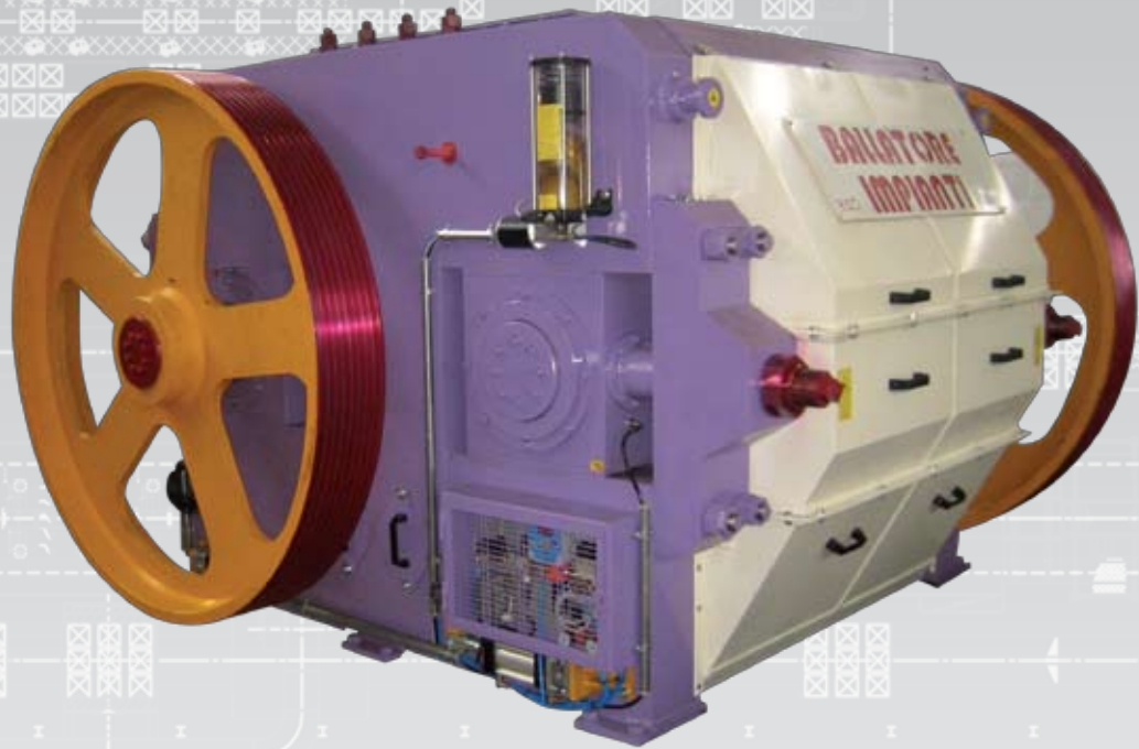
LAMINATOIO serie LM - COD. F-03 ROLLER MILL LM series / LAMINOIR série LM
