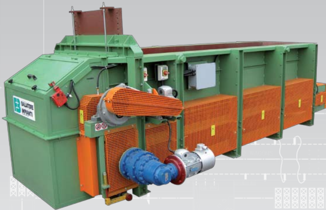
DOSATORE A TAPPETO IN GOMMA serie CRG - COD. F-01-20/22 RUBBER BELT BOX FEEDER CRG serie / DOSEUR À TAPIS EN CAOUTCHOUC série CRG
