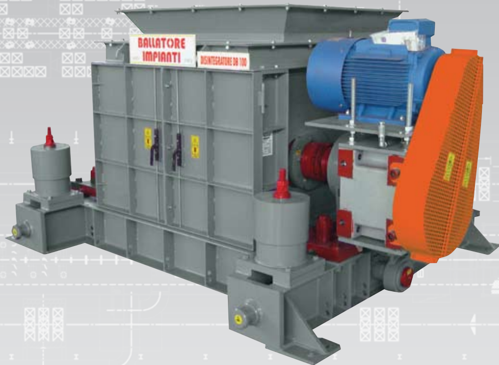
DISINTEGRATORE A BARRETTE serie DB - COD. F-02-03 BAR CRUSHER DB series - COD. F-02-03 / DÉSINTÉGRATEUR À BARRETTES série DB - COD. F-02-03
