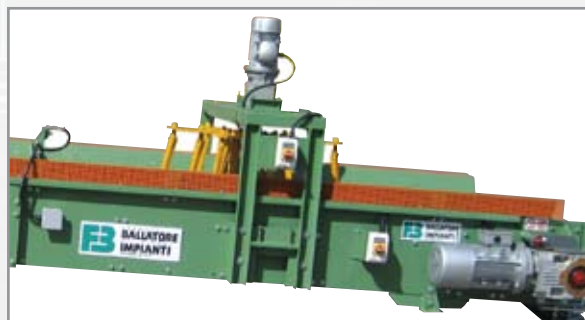
NASTRO INCERNIERATO / TILTING CONVEYOR END CONVOYEUR FLOTTANT SUR PARTIE FINAL
